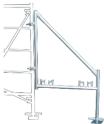
Outrigger
