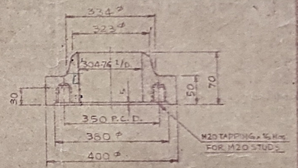
DETAIL B MATL: SA 182 F 316
