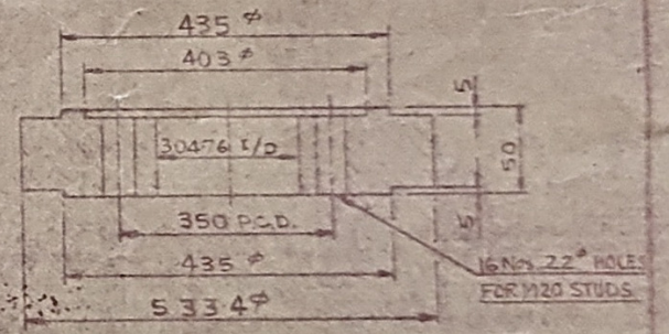
DETAIL C MATL: SA 182 F 316
