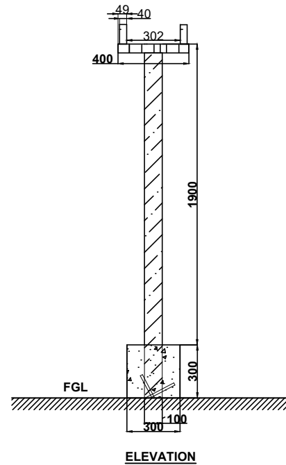
ELEVATION
